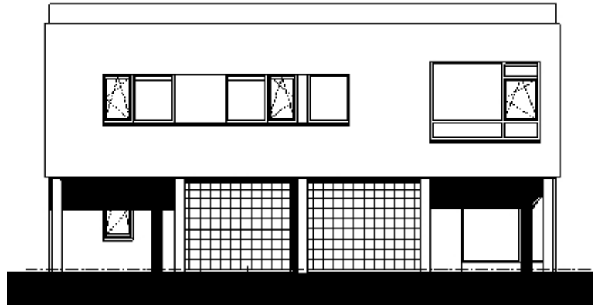
Voorgevel villa
