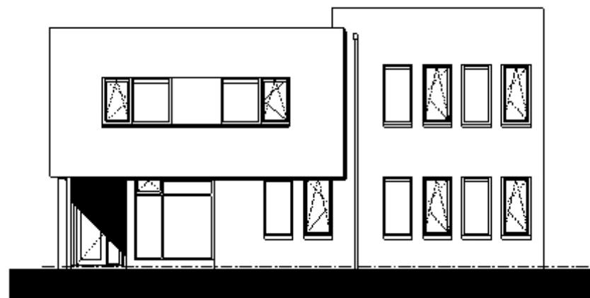
Zijgevel villa
