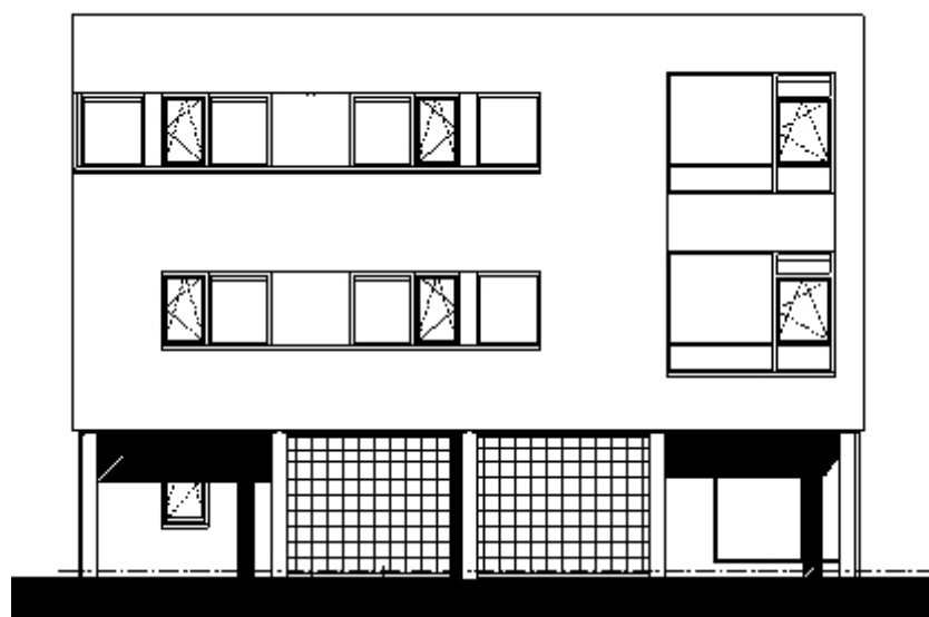
Voorgevel Poortgebouw
