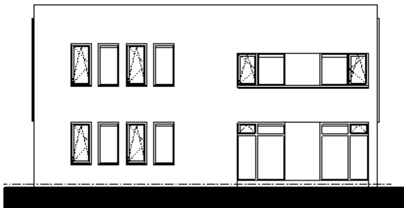
Achtergevel villa
