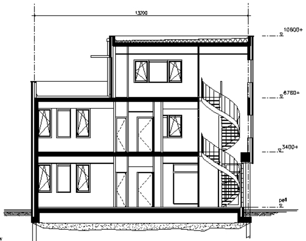
Doorsnede Poortgebouw
